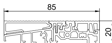
поріг TS88510-FL+TSA8851
