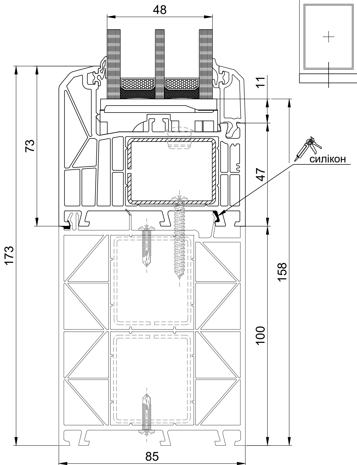
СХЕМА 850165 РАМА 73 мм 180204 розширювач 100 мм
