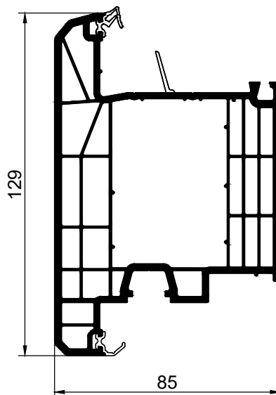
850465 стулка дверна 129мм
