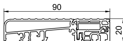
поріг greenteQ TB90 AS
