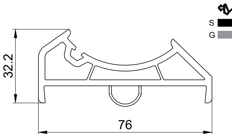
551465 адаптер еркера
