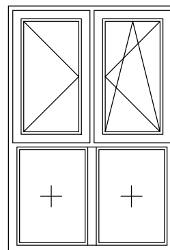
двостулкове поворотне/ поворотно - відкидне відкривання з глухим склінням нижньої частини
