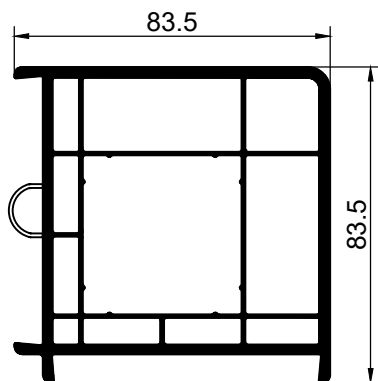
551665 з'єднувач 90°
