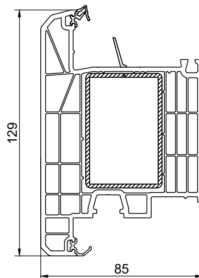
850465 стулка дверна 129мм
