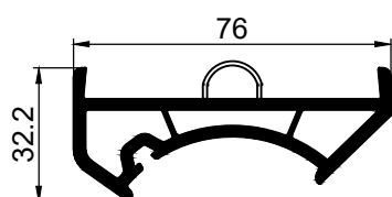
551465 адаптер еркера
