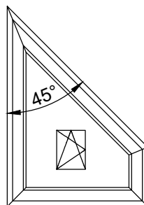
поворотно - відкидне відкидне трапецієвидне вікно
