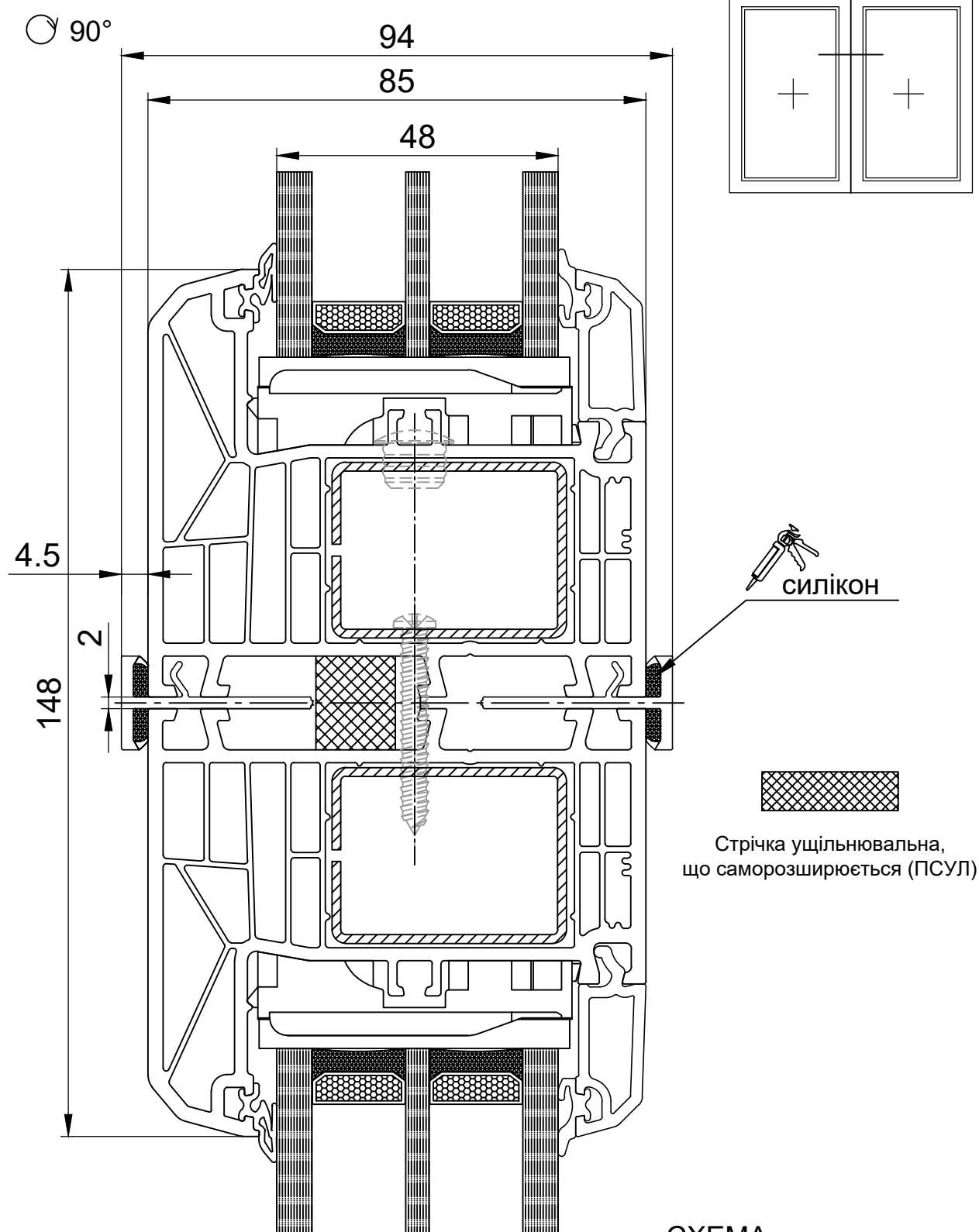
СХЕМА 850165 РАМА 73 мм 552300 з'єднувач Н-подібний 850165 РАМА 73 мм
