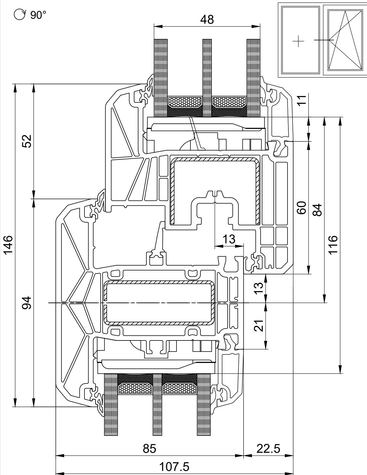
СХЕМА 850365 ІМПОСТ 94 мм 850265 СТУЛКА 86 мм
