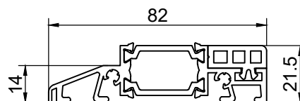
поріг алюмінієвий анодований (з термомостом)
