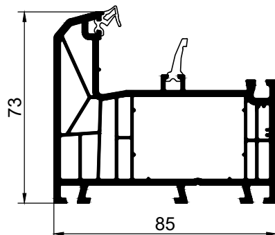
850165 рама 73мм
