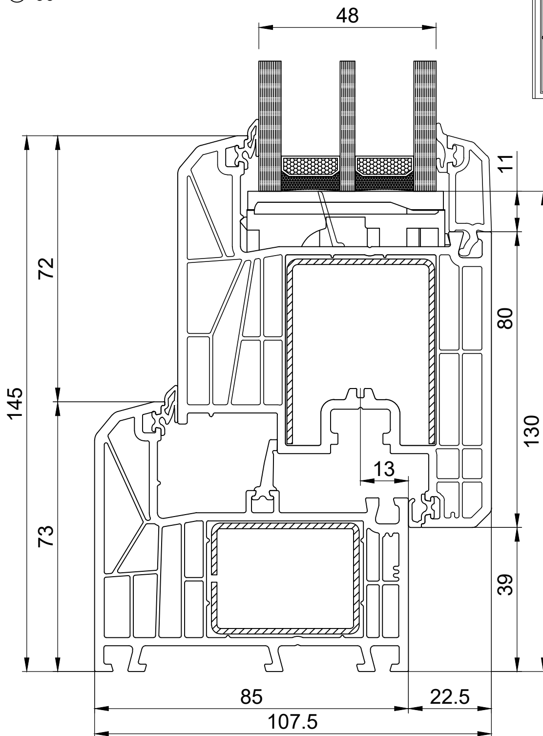
СХЕМА 850165 РАМА 73 мм 850565 СТУЛКА ДВЕРНА 106 мм
