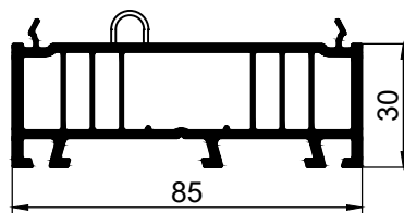
851765 розширювач 30мм
