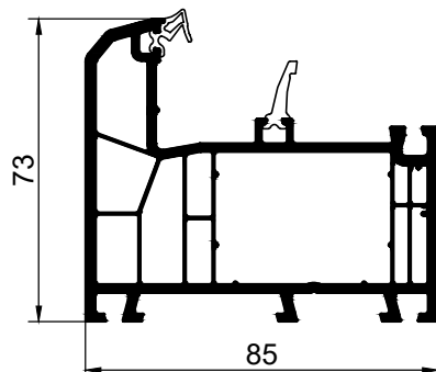
852165 рама 73мм
