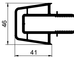
111965 з'єднувач статичний
