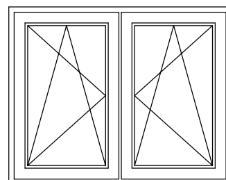
двостулкове імпостне поворотно - відкидне відкривання
